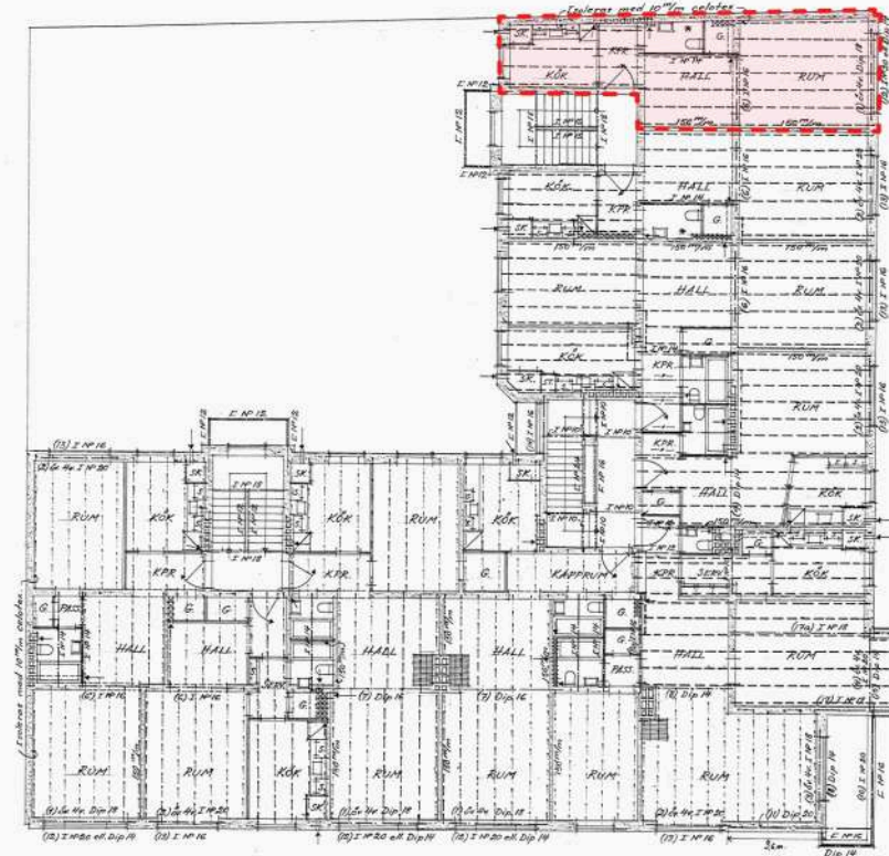
PLAN AV 2-DRA, 3-DJE & 4-DE VÅN.
